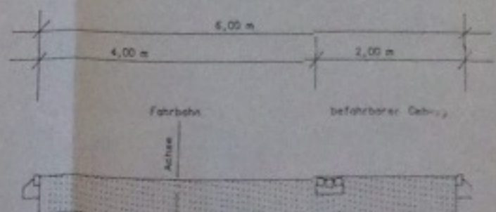
Regelprofil Erschließungsstraße
