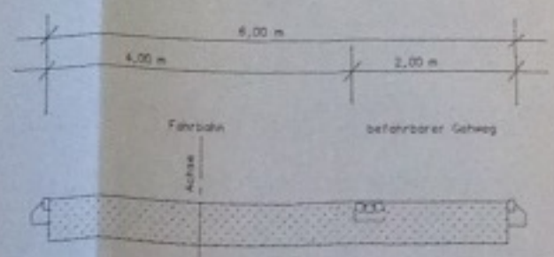
Regelprofil Erschließungsstraße
